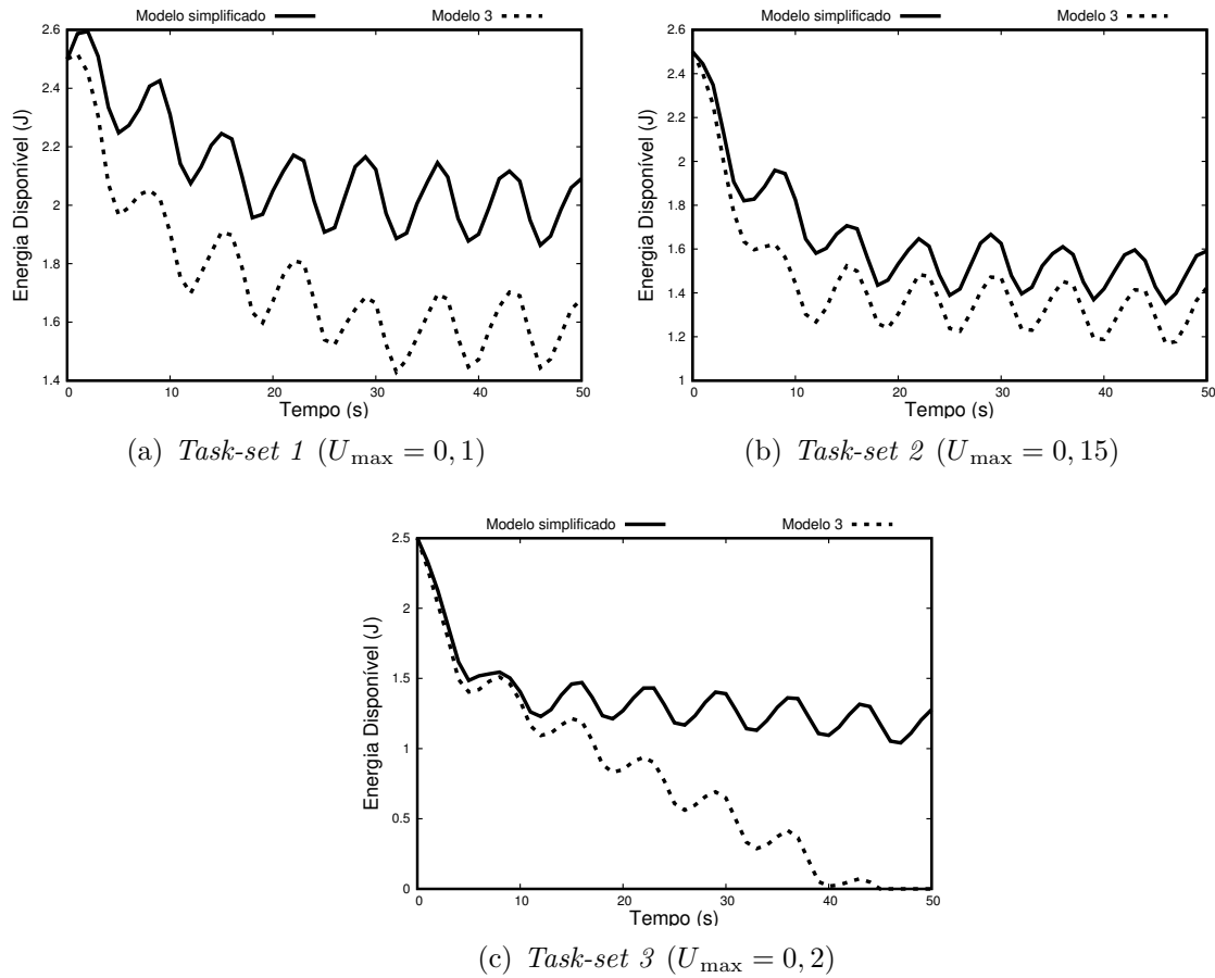
Figura 27 – Comparativo entre o modelo simplificado e o modelo 3.
