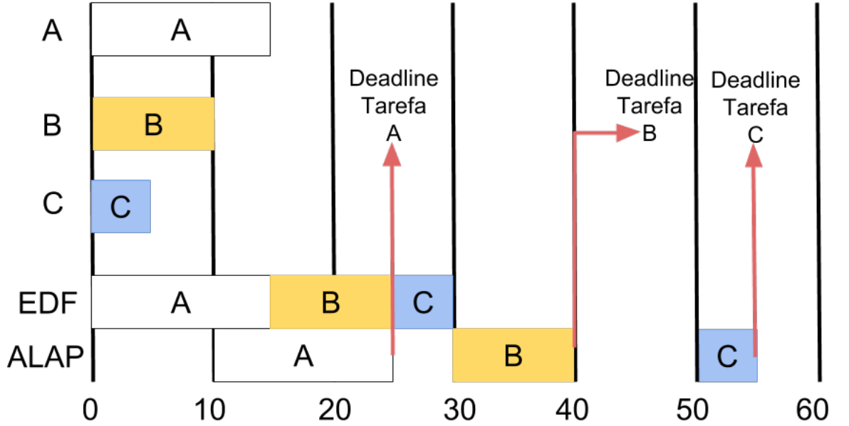
Figura 10 – Comparativo EDF X ALAP
