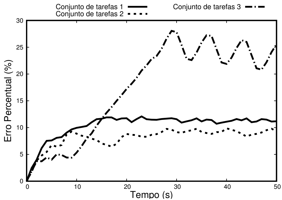
Figura 35 – Erro percentual por segundo (modelo complexo)
