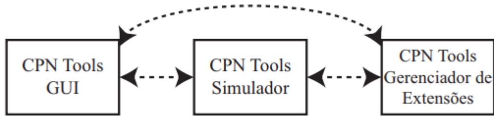
Figura 12 – Arquitetura do CPN Tools 4.
