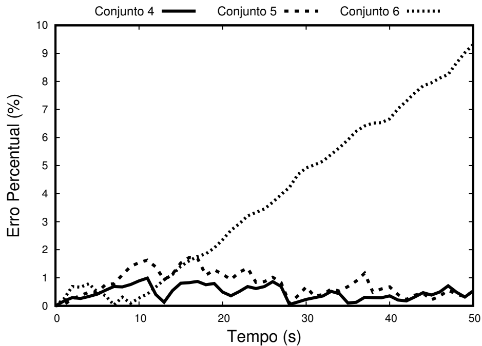
Figura 32 – Erro percentual por segundo (modelo 4)
