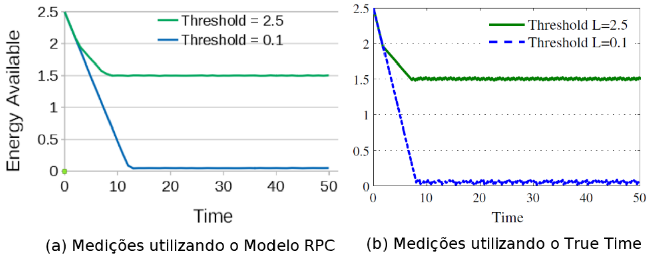
Figura 21 – Comparativo entre o SECE-CPN e o TrueTime.
