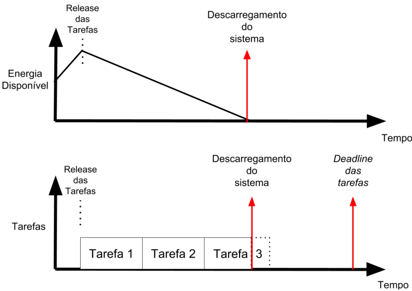
(a) Escalonamento sequencial mais rápido possível
