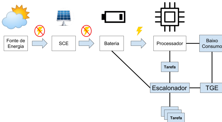
(b) Estado de energia escassa
