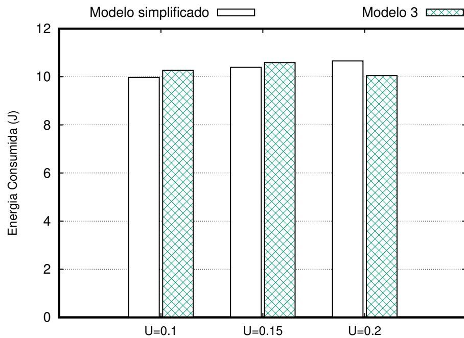
Figura 29 – Consumo energético total do sistema (modelo 3)
