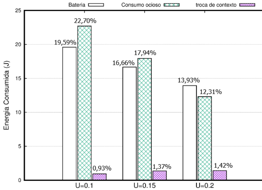
Figura 37 – Energia negligenciada pelas simplificações em relação ao consumo total.
