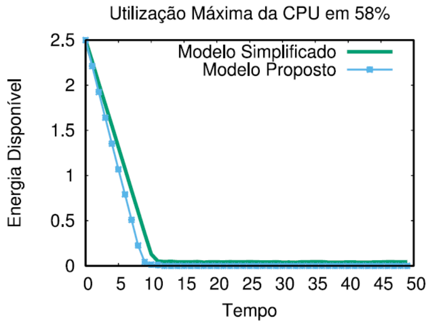
Figura 23 – Energia disponível utilizando o conjunto de tarefas 2
