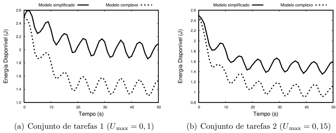
Figura 34 – Comparativo entre o modelo simplificado e o modelo 5.
