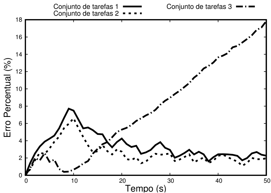
Figura 25 – Erro de medição por segundo (Modelo 2).
