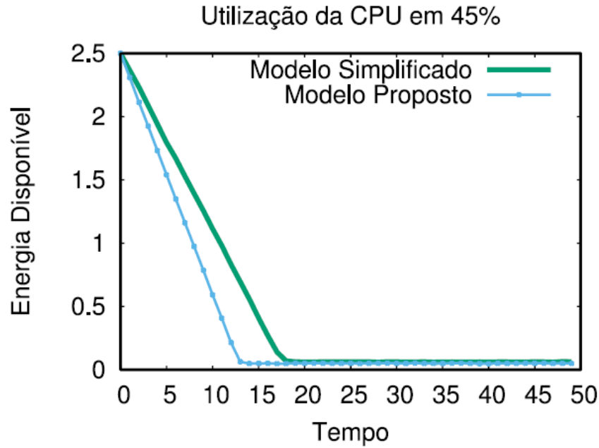
Figura 22 – Energia disponível utilizando o conjunto de tarefas 1
