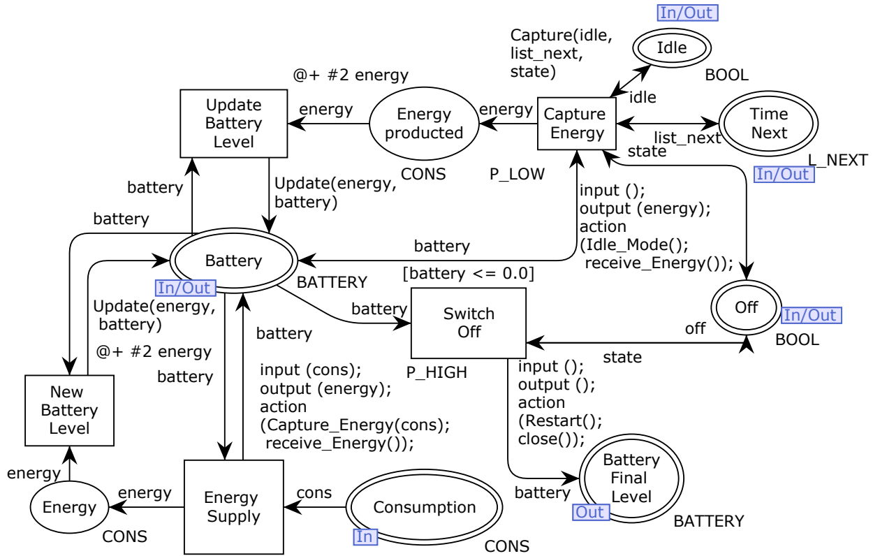
Figura 20 – Subpágina Energy Harvesting
