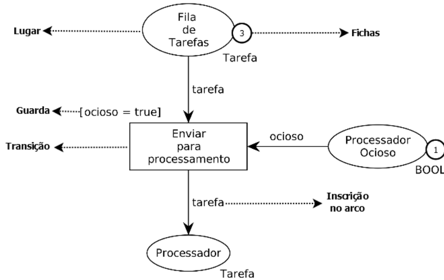
Figura 11 – Estrutura Típica de uma RPC
