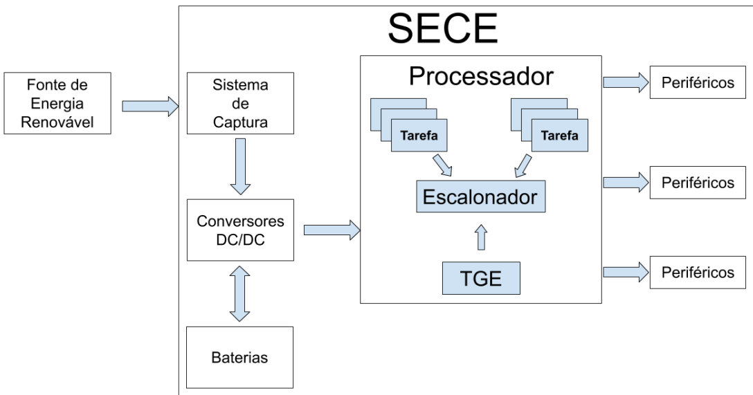
Figura 3 – Arquitetura típica para SECEs
