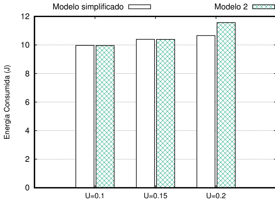
Figura 26 – Consumo energético total do sistema (modelo 2).
