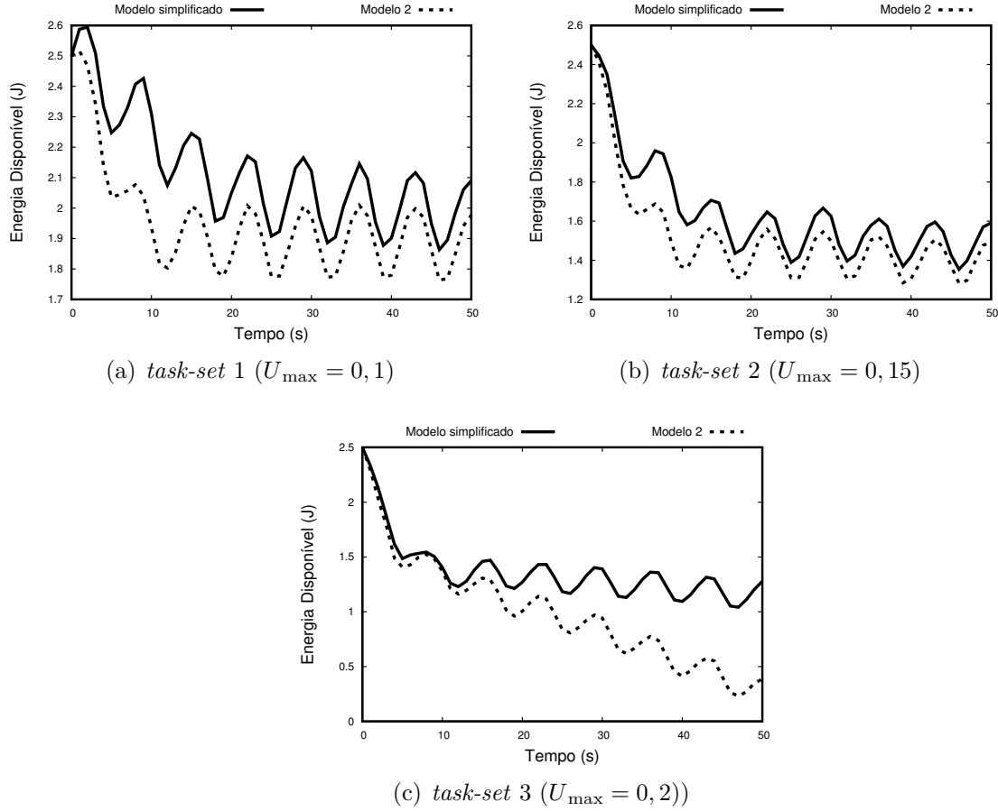
Figura 24 – Comparativo entre o modelo simplificado e o modelo 2.
