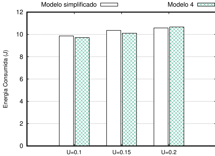
Figura 33 – Consumo energético do sistema (modelo 4)
