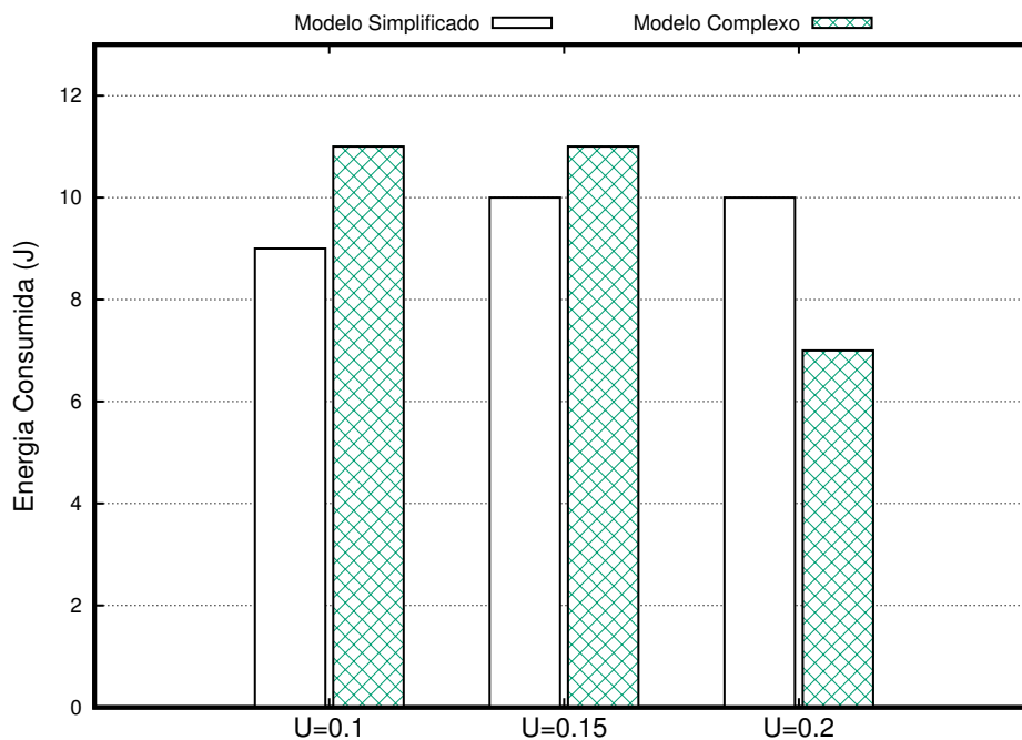
Figura 36 – Consumo energético total do sistema (modelo 5)
