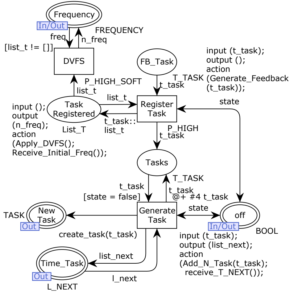
Figura 17 – Subpágina Task Generator
