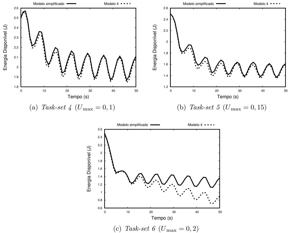
Figura 31 – Comparativo entre o modelo simplificado e o modelo 4 utilizando os novos conjuntos de tarefas.
