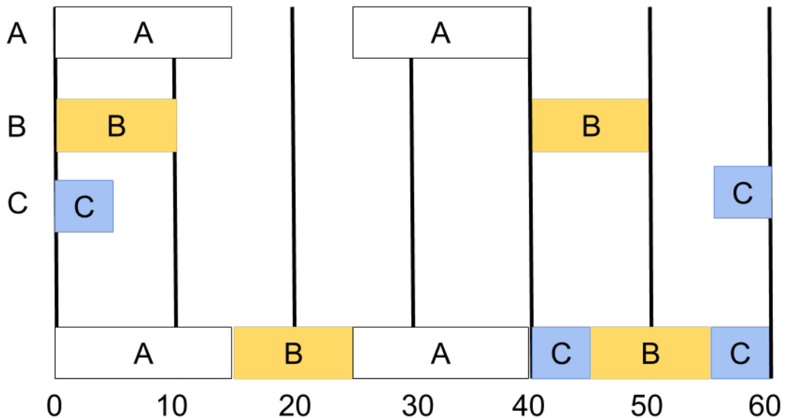
Figura 9 – Escalonamento segundo o algoritmo EDF
