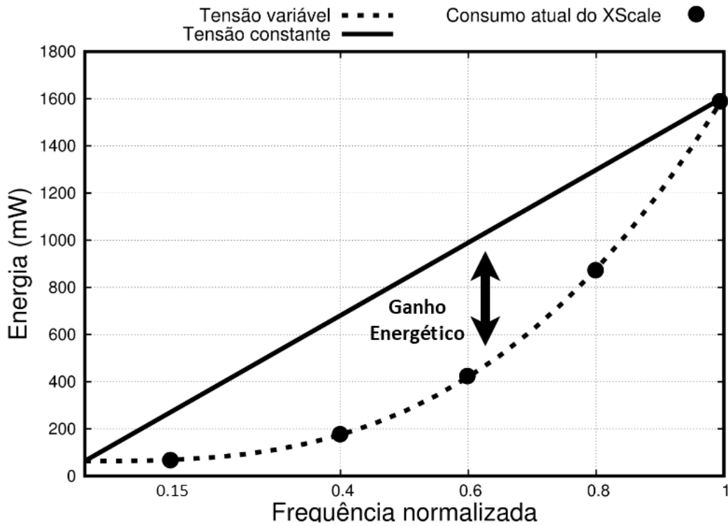
Figura 4 – Ganho energético alcançado com o uso de DVFS.
