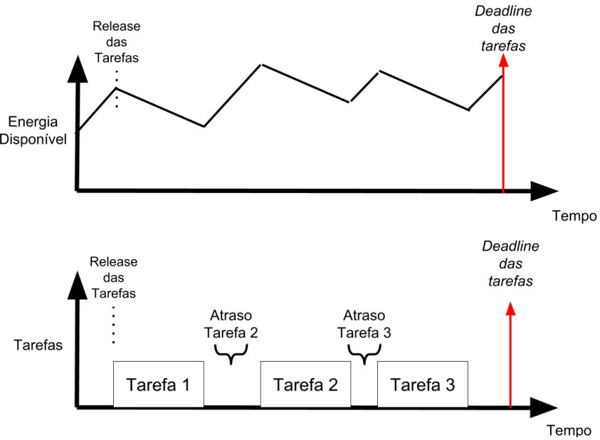
(b) Escalonamento com atraso
