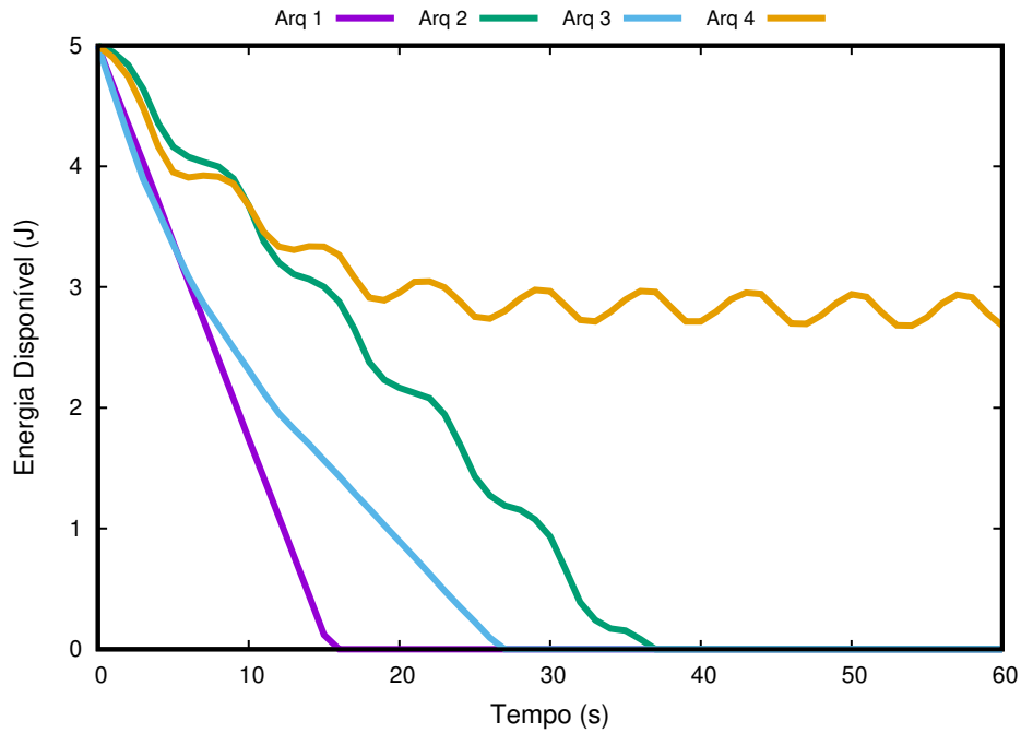
Figura 8 – Consumo energético de um mesmo sistema sob arquiteturas diferentes.
