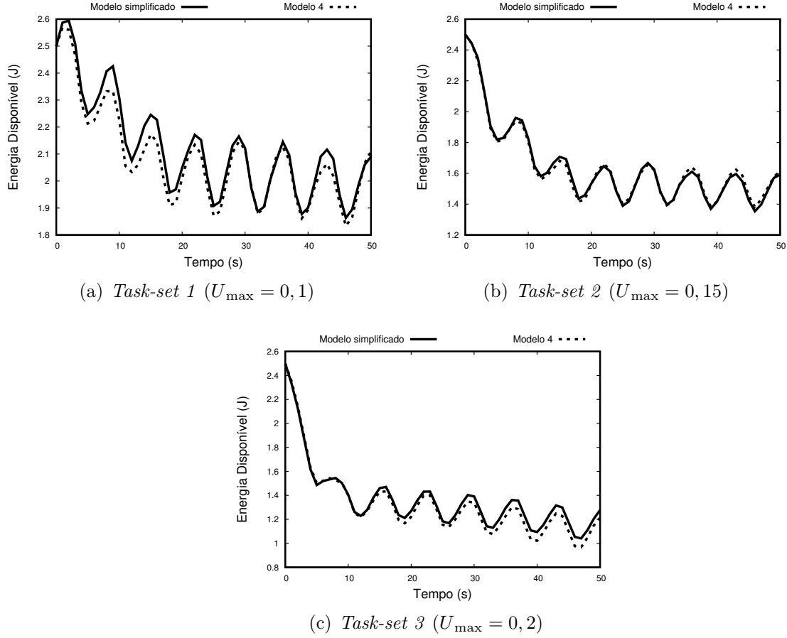
Figura 30 – Comparativo entre o modelo simplificado e o modelo 4.
