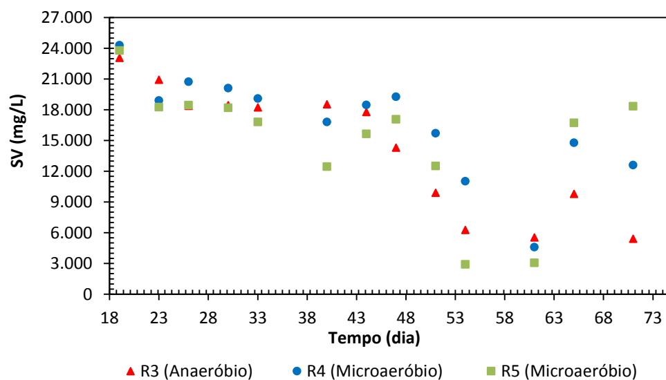
Figura 35 - Remoção de sólidos voláteis (SV) de R3, R4 e R5 durante o experimento 2 semicontínuo
