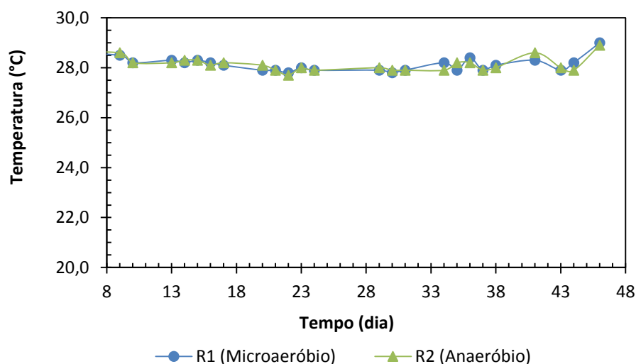
Figura 23 -Variação da temperatura dos reatores R1 e R2 em batelada
