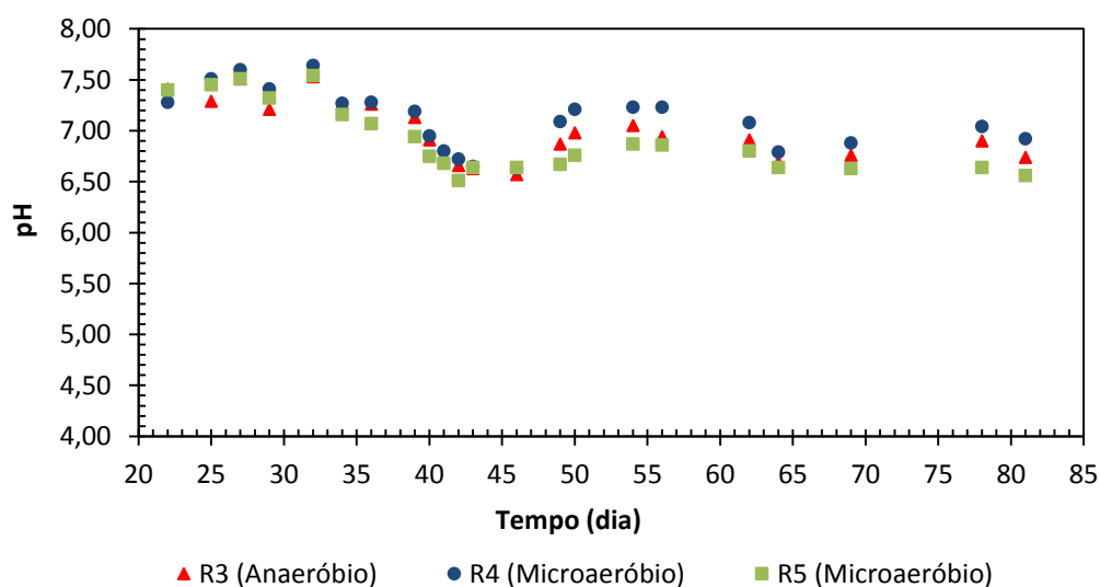
Figura 25 - Variação de pH dos reatores R3, R4 e R5 no experimento 3 semicontínuo
