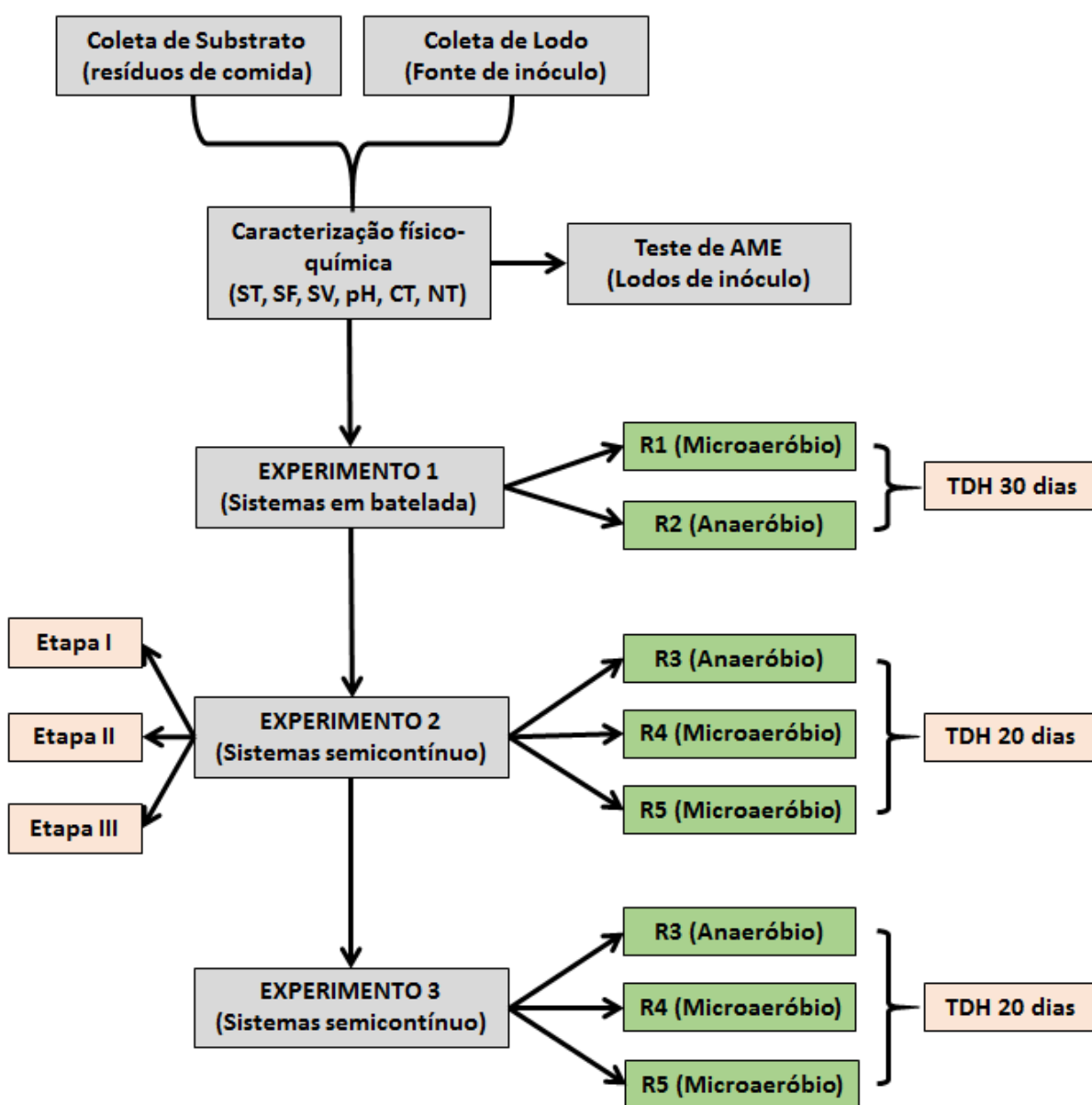
Figura 2 - Fluxograma do procedimento experimental da pesquisa
