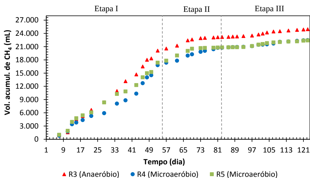
Figura 37 - Volume acumulado de metano em R3, R4 e R5 durante o experimento 2
