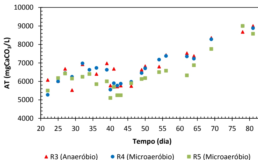
Figura 28 - Variação de alcalinidade total de R3, R4 e R5 durante o experimento 3 semicontínuo
