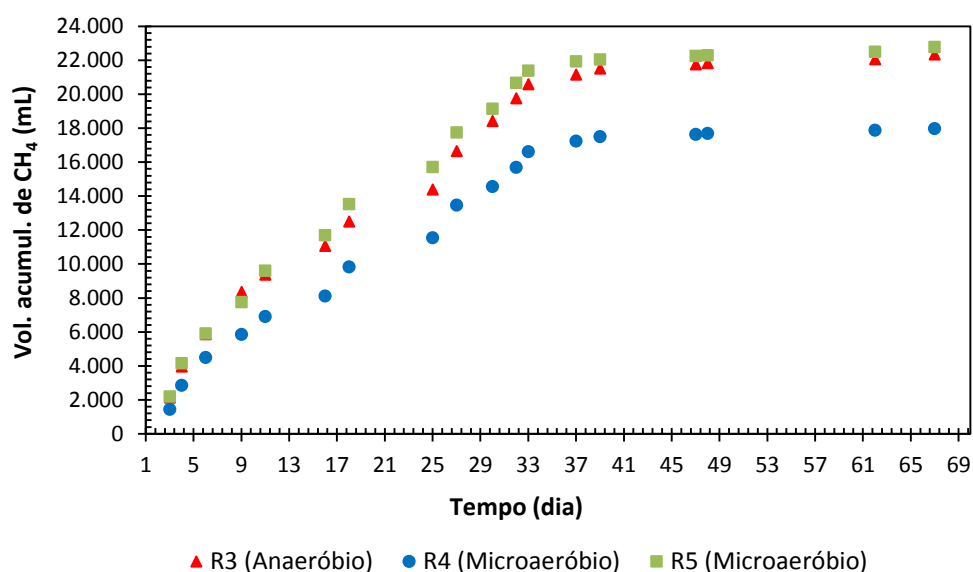
Figura 39 - Volume acumulado de metano em R3, R4 e R5 durante o experimento 3
