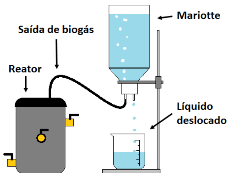
Figura 12 - Representação esquemática do sistema de medição do biogás nos reatores
