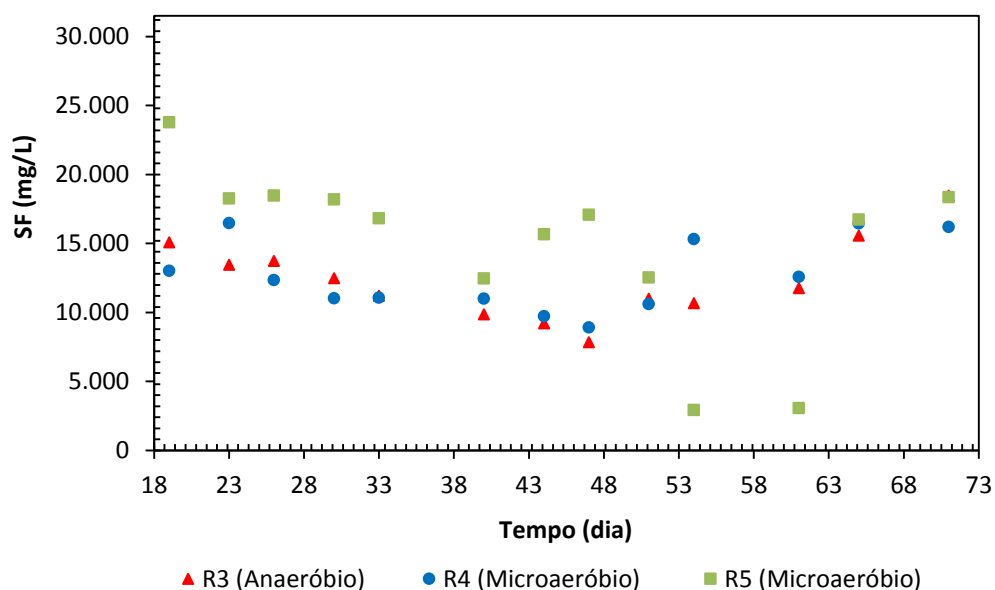
Figura 34 - Concentração de sólidos fixos (SF) de R3, R4 e R5 durante o experimento 2 semicontínuo
