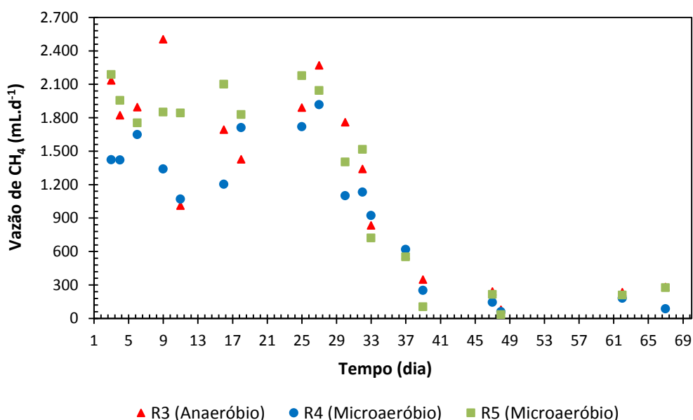
Figura 38 - Vazão de metano nos reatores R3, R4 e R5 durante o experimento 3
