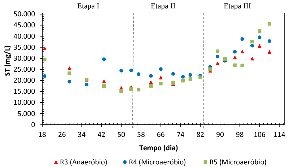
Figura 30 - Remoção de sólidos totais (ST) de R3, R4 e R5 durante o experimento 2 semicontínuos
