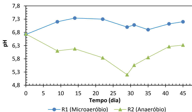
Figura 19 - Variação temporal do pH nos reatores R1 e R2 em batelada
