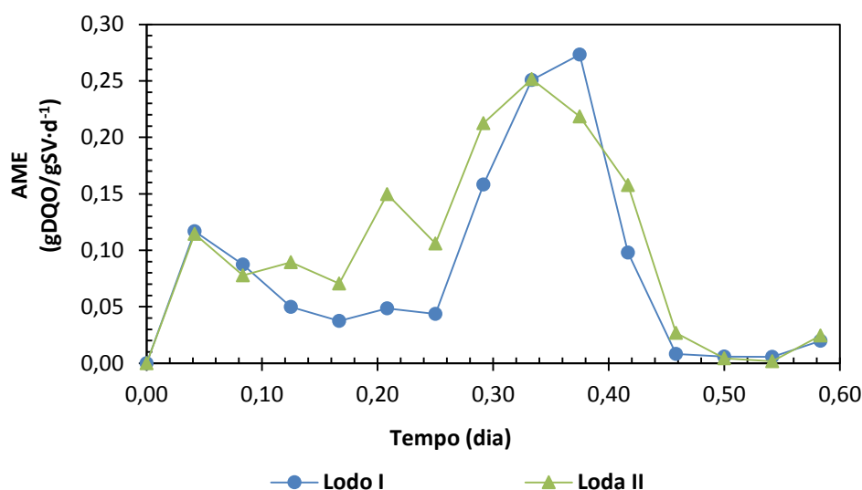
Figura 18 - Atividade metanogênica específica dos lodos 1 e 2
