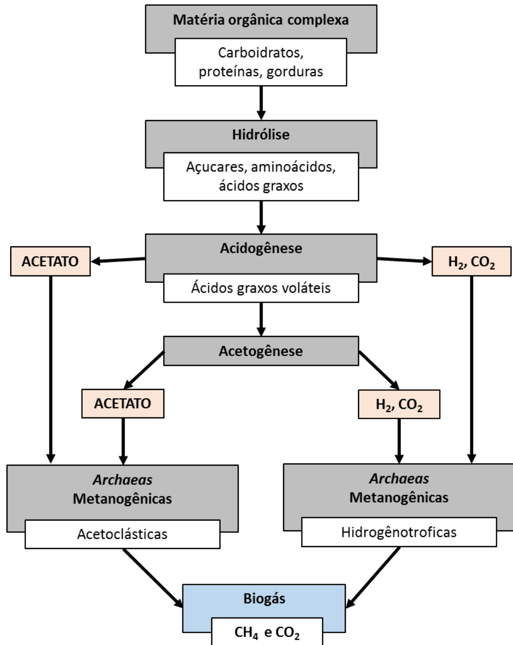
Figura 1 - Rotas metabólicas e microrganismos da digestão anaeróbia
