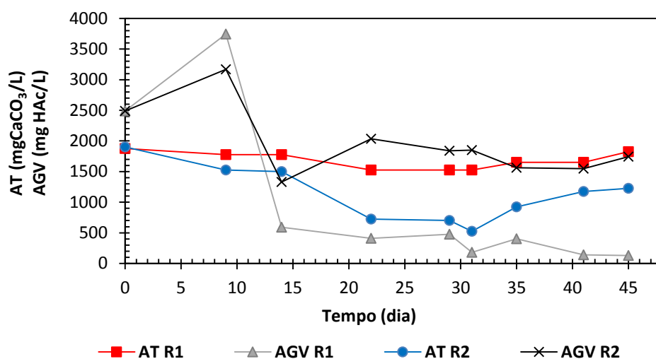
Figura 20 - Variação temporal de AT e AGV de R1 e R2
