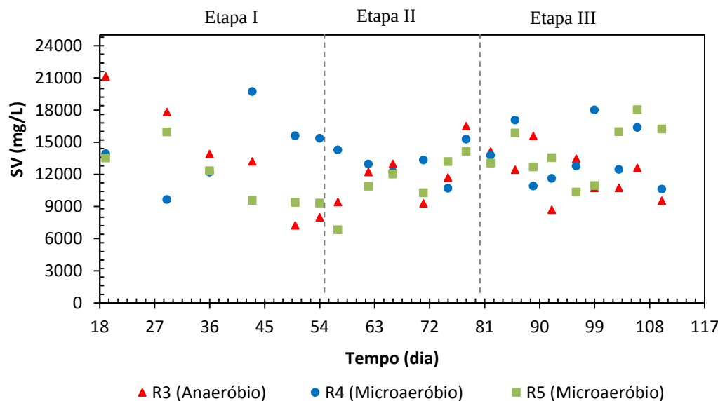
Figura 32 - Remoção de sólidos voláteis (SV) de R3, R4 e R5 durante o experimento 2 semicontínuo
