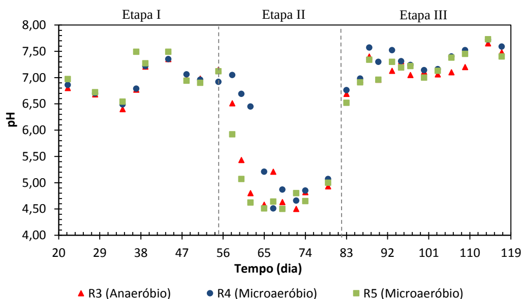
Figura 24 - Variação de pH dos reatores R3, R4 e R5 no experimento 2 semicontínuo
