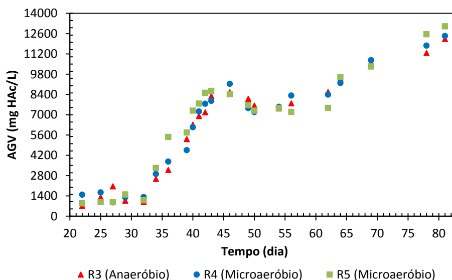
Figura 29 - Produção de ácidos graxos voláteis (AGV) durante o experimento 3 semicontínuo
