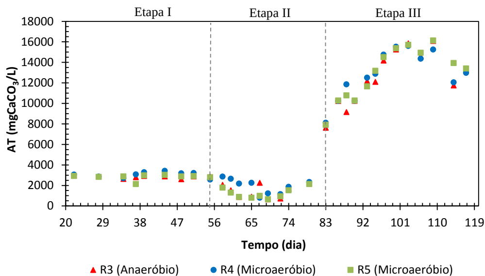
Figura 26 - Variação de alcalinidade total de R3, R4 e R5 durante o experimento 2 semicontínuo
