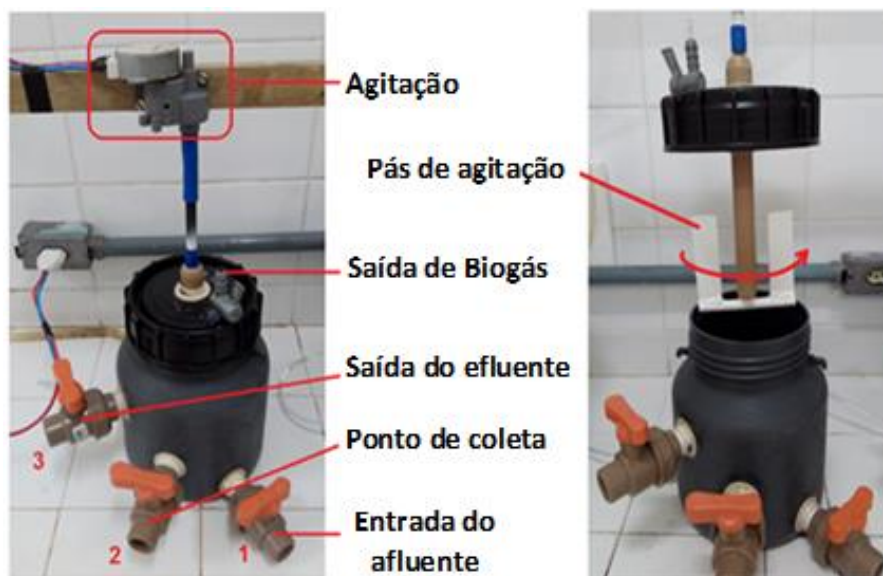
Figura 9 - Biorreator anaeróbio semicontínuo e sistema de agitação
