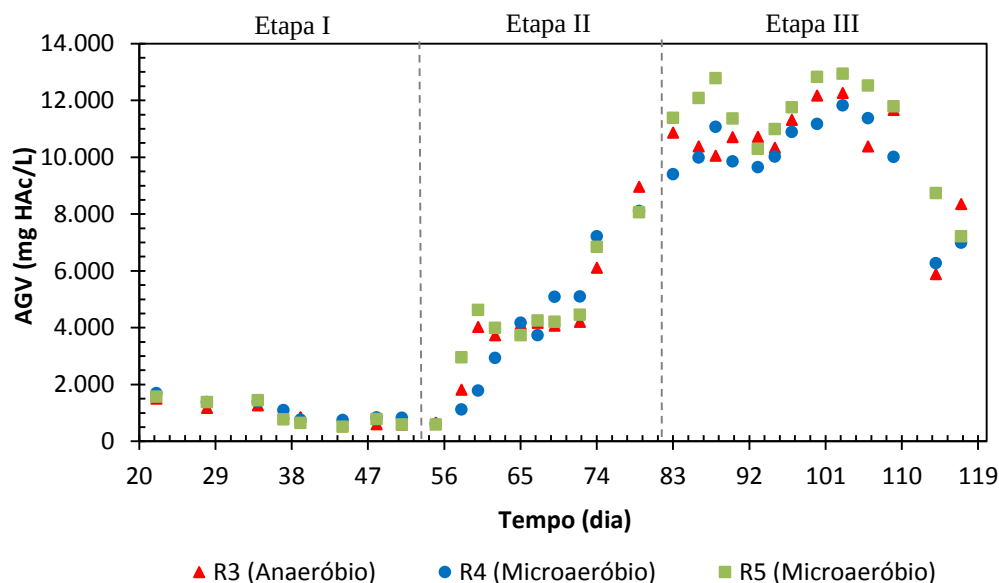
Figura 27 - Produção de ácidos graxos voláteis (AGV) durante o experimento 2 semicontínuo
