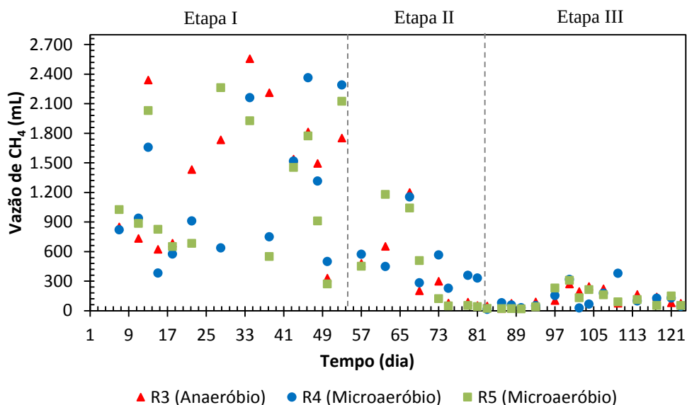
Figura 36 - Vazão de metano nos reatores R3, R4 e R5 durante o experimento 2
