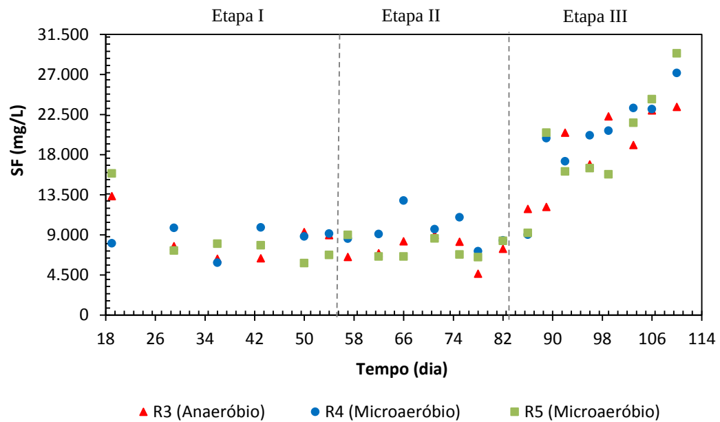
Figura 31 - Concentração de sólidos fixos (SF) de R3, R4 e R5 durante o experimento 2 semicontínuo
