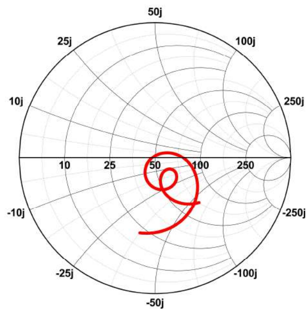
Figura 57: Carta de Smith para DRA com \epsilon_r = 17 e furo central de 2.25 mm
