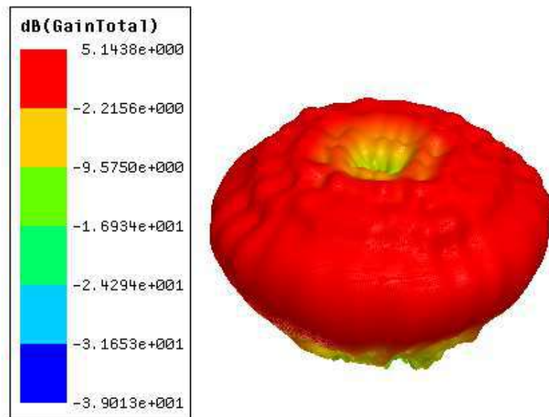
Figura 38: Diagrama de radiação 3D da DRA para com permissividade dielétrica \epsilon_r = 17 para primeira frequência de ressonância
