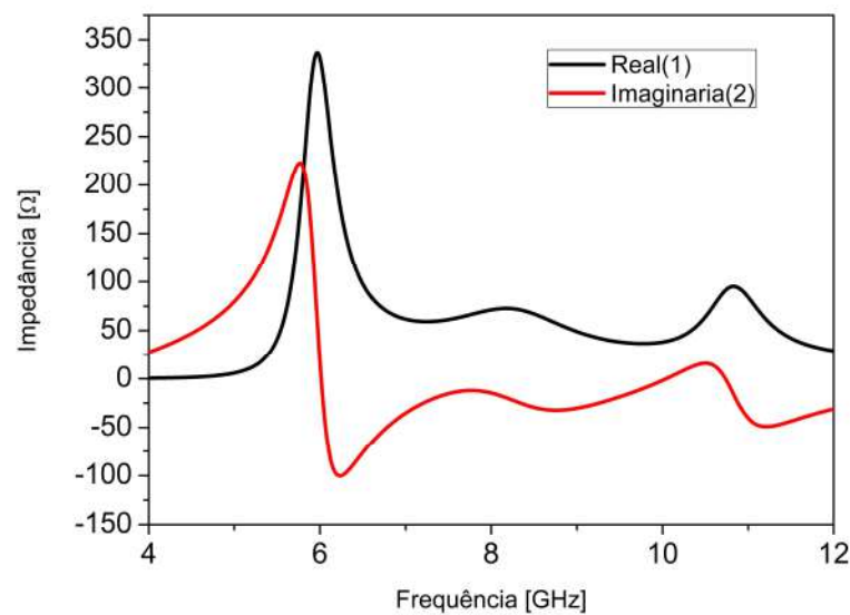
Figura 35: Impedância real e imaginária para DRA com \epsilon_r = 17
