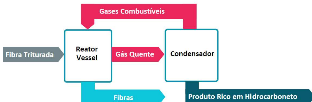
Figura 24 – Diagrama de processo da pirólise.
