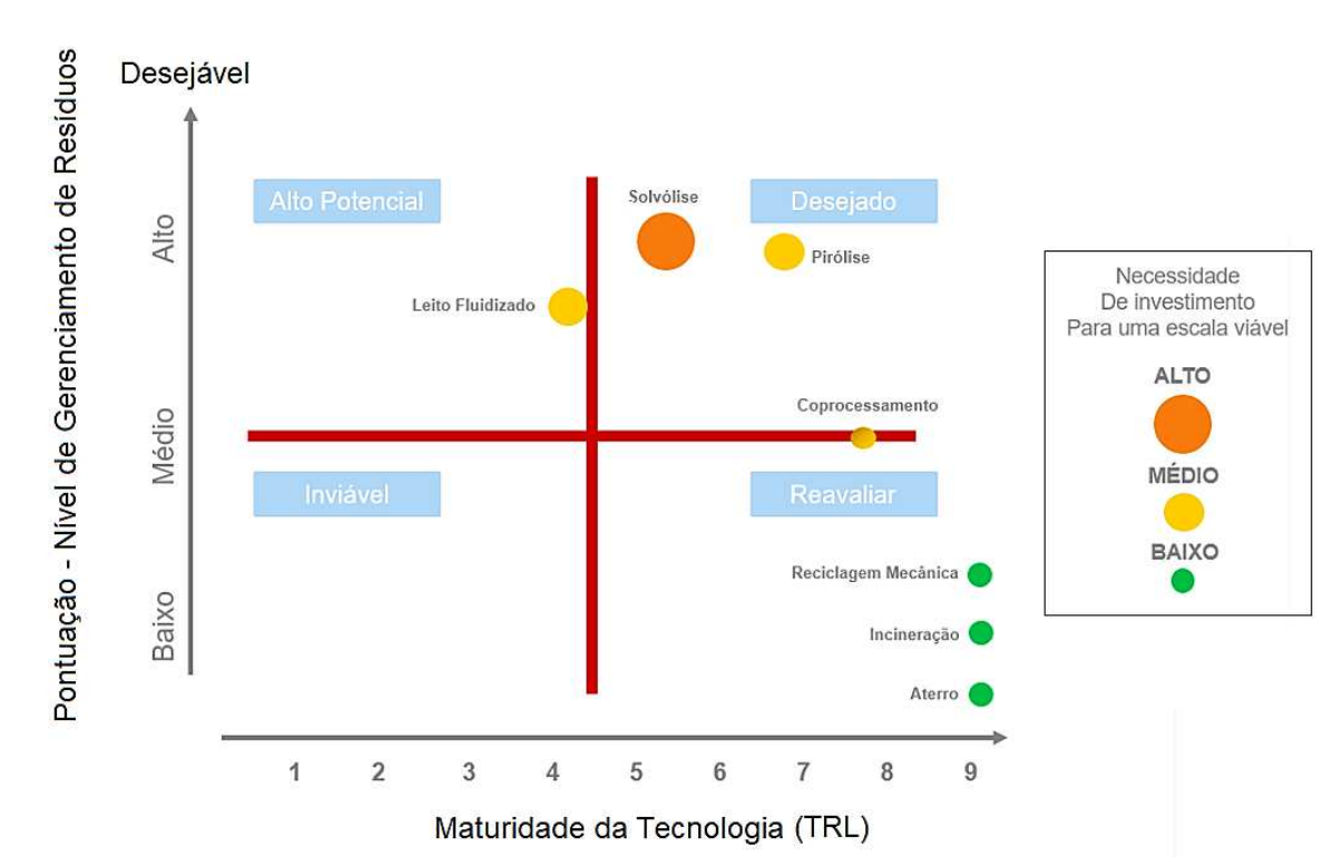
Figura 33 – TRL de diferentes métodos de reciclagem.
