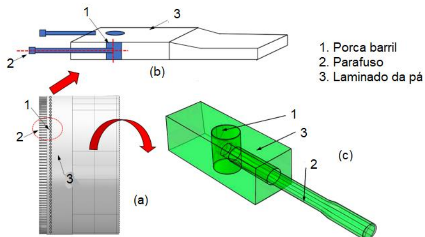
Figura 15 - (a) Típica estrutura de uma raiz de pá eólica com componentes mecânicos; (b) (c) Conexões mecânicas entre porca barril e parafuso.
