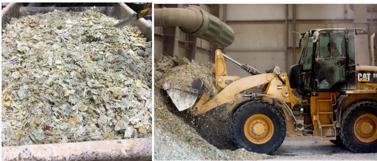
Figura 41 – Resíduo de pá triturada e armazenamento de resíduos triturados provenientes de pás eólicas.
