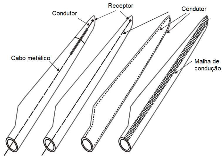
Figura 16: Sistema de proteção contra descargas atmosféricas.
