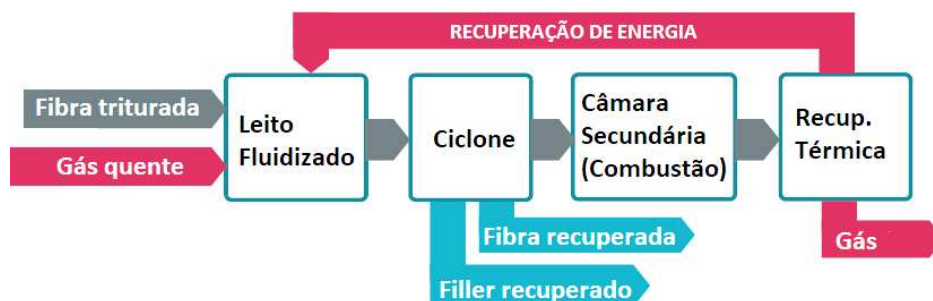
Figura 25 – Diagrama de processo do leito fluidizado.
