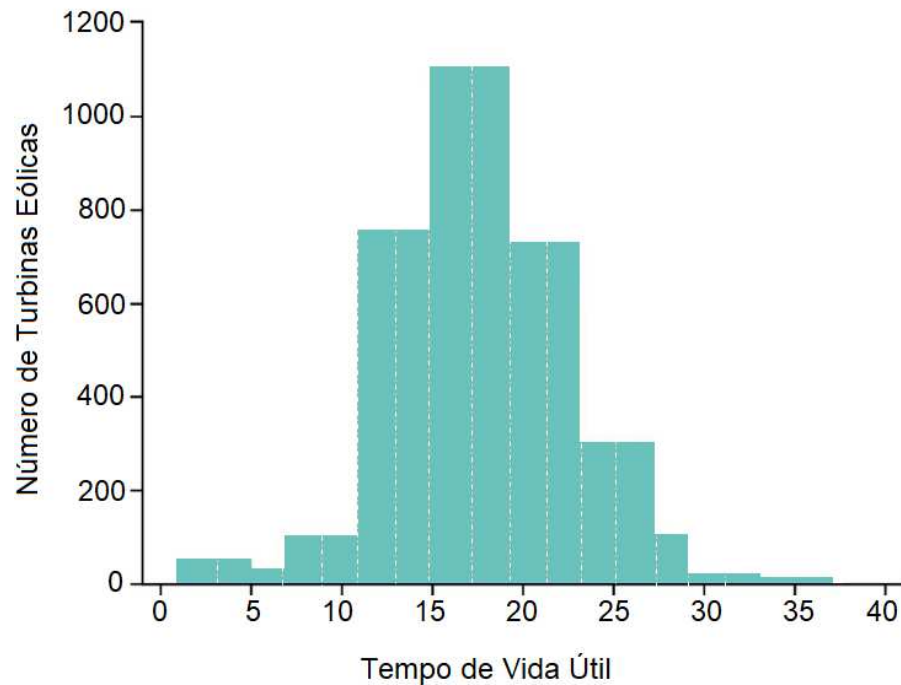
Figura 47 - Distribuição histórica de fim de vida útil de turbinas eólicas
