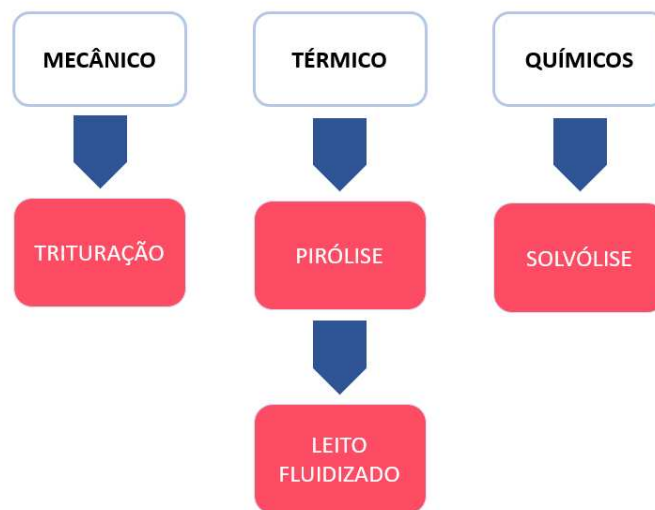
Figura 22 – Diagrama dos principais processos para reciclagem de pás de turbinas eólicas.
