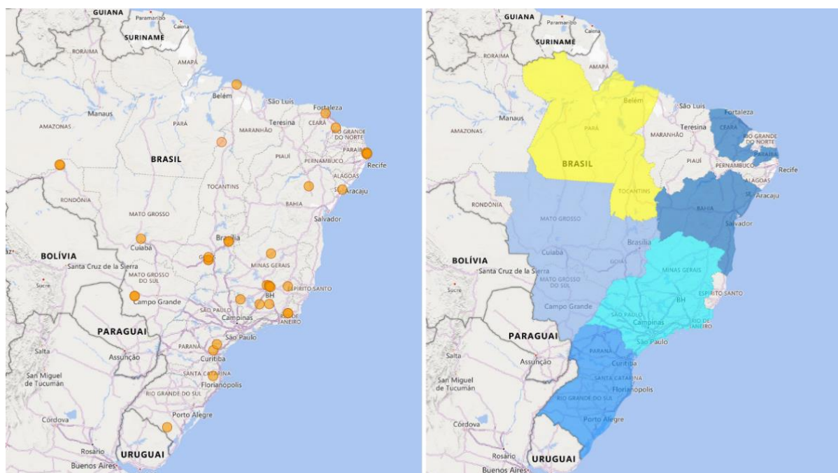
Figura 53 – Mapeamento de plantas de coprocessamento de resíduos no Brasil.
