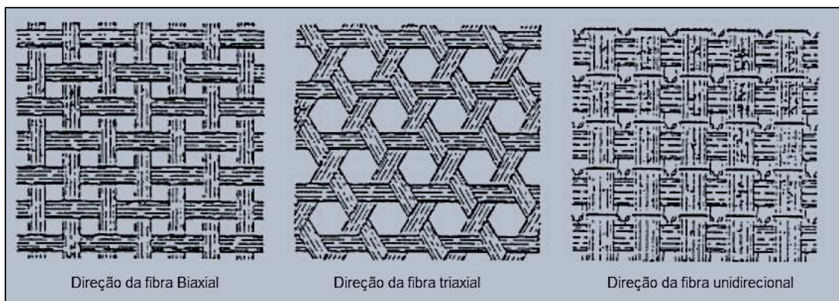
Figura 12 - Orientação de fibras
