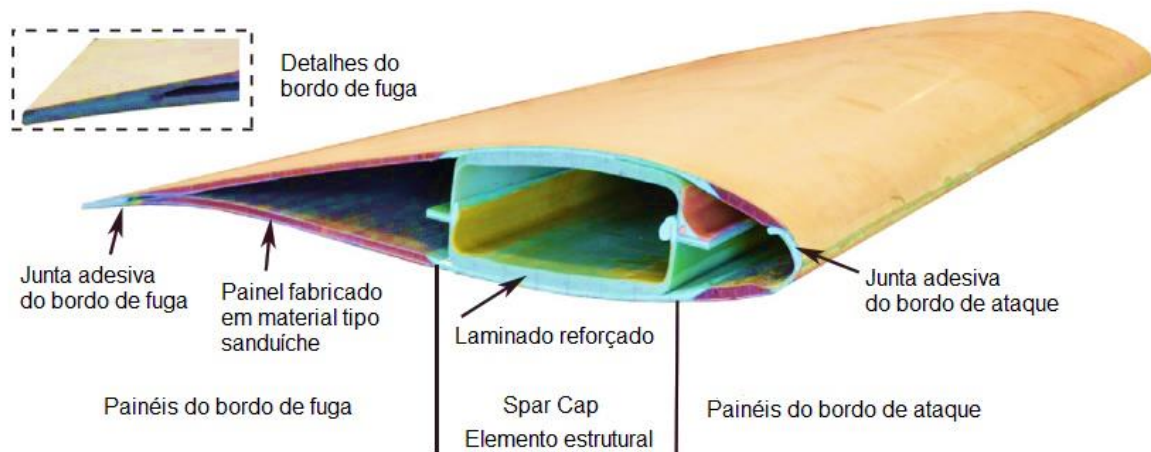
Figura 7 - Seção transversal de uma pá eólica.
