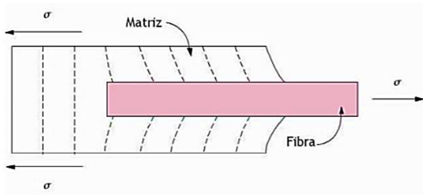
Figura 10 - Deformação na matriz circundante de uma fibra submetida a uma carga de tração segue um padrão.
