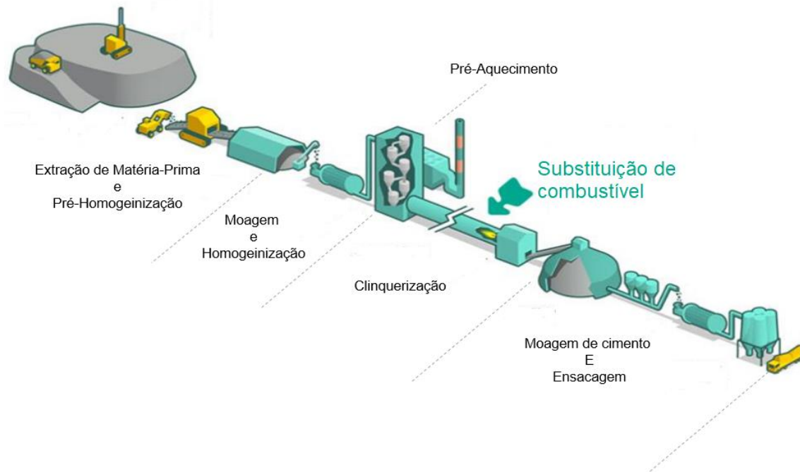
Figura 35 – Fluxograma de fábrica de cimento.
