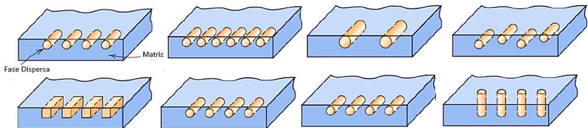
Figura 9 - Esquema das possíveis distribuições do reforço no compósito em função da concentração, forma, distribuição e orientação do reforço.
