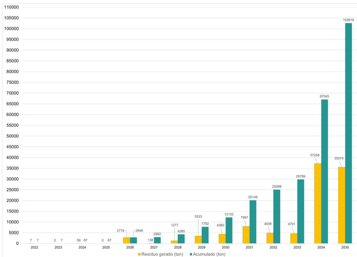
Figura 52 – Estimativa da quantidade de resíduos (tons) provenientes de pás eólicas gerados pelo seu descomissionamento (Dados em toneladas).
