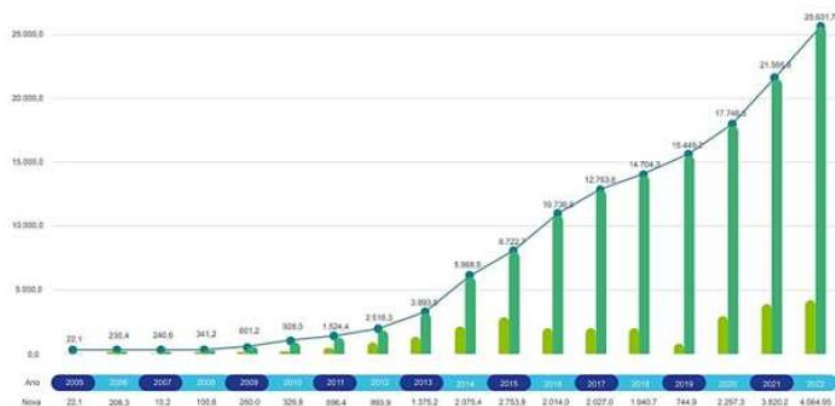
Figura: Expansão da capacidade instalada de turbinas eólica no Brasil. Dados em MW (Fonte: ABEEólica, 2022)
