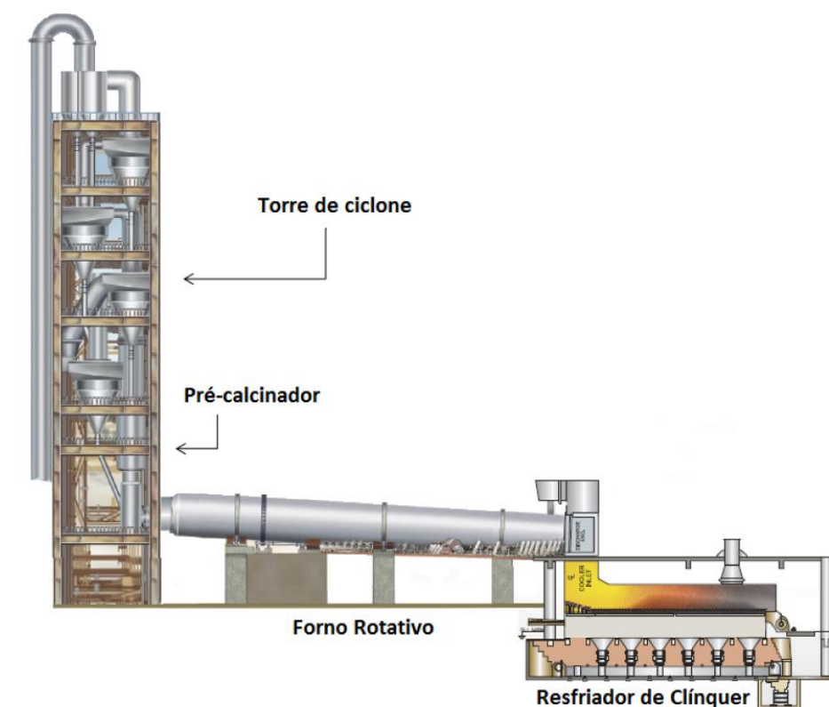
Figura 37 - Conjunto do pré-aquecedor, pré-calcinador e forno rotativo de clínquer.
