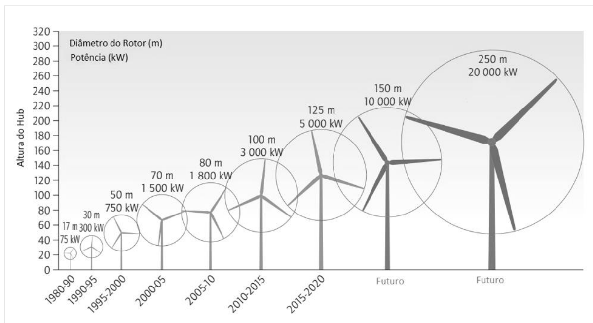
Figura 48 – Evolução histórica de tamanho de turbinas eólicas.
