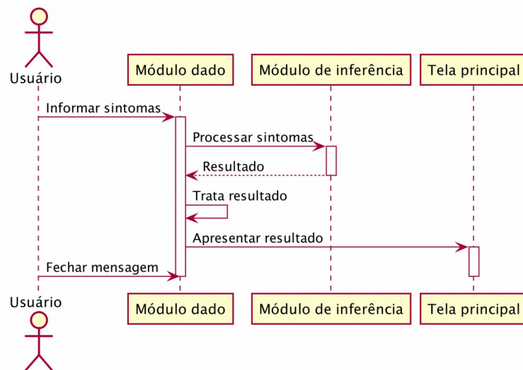
Figura 18 – Diagrama de Sequência para módulo service.dado .
