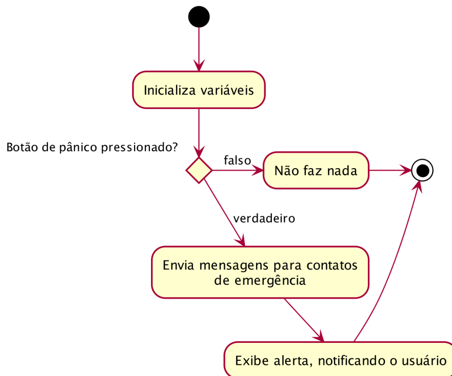
Figura 32 – Diagrama de Atividades para módulo service.panicbutton .
