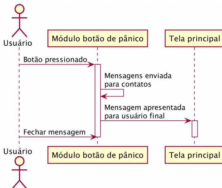
Figura 19 – Diagrama de Sequência para módulo service.panicbutton .
