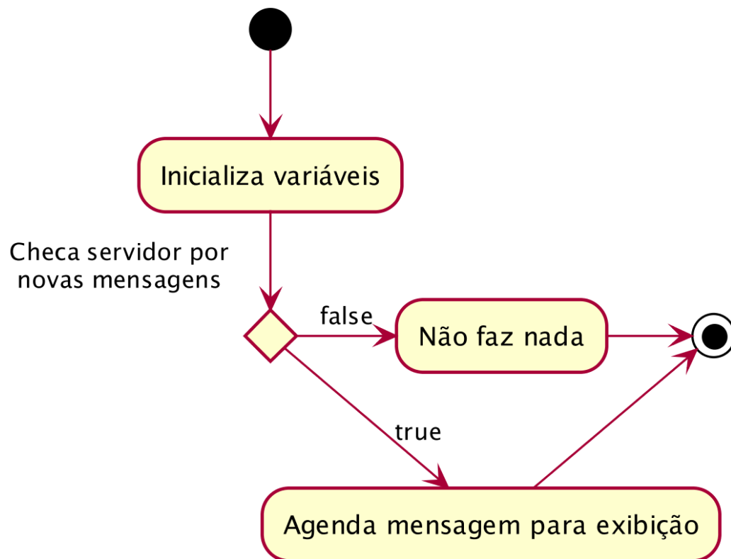
Figura 28 – Diagrama de Atividades para módulo service.notification .
