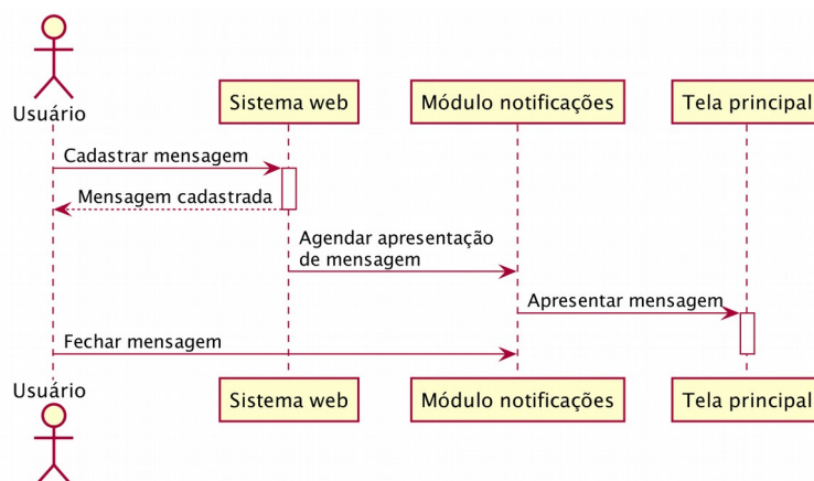
Figura 16 – Diagrama de Sequência para módulo service.notification . Alerta do tipo caixa de diálogo.
