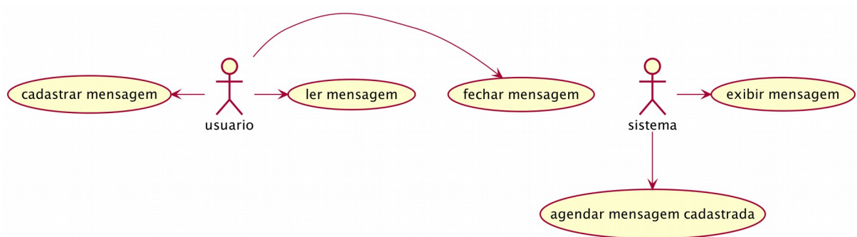
Figura 27 – Diagrama de Caso de Uso para módulo service.notification .
