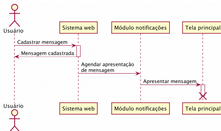
Figura 17 – Diagrama de Sequência para módulo service.notification . Alerta do tipo pop-up .
