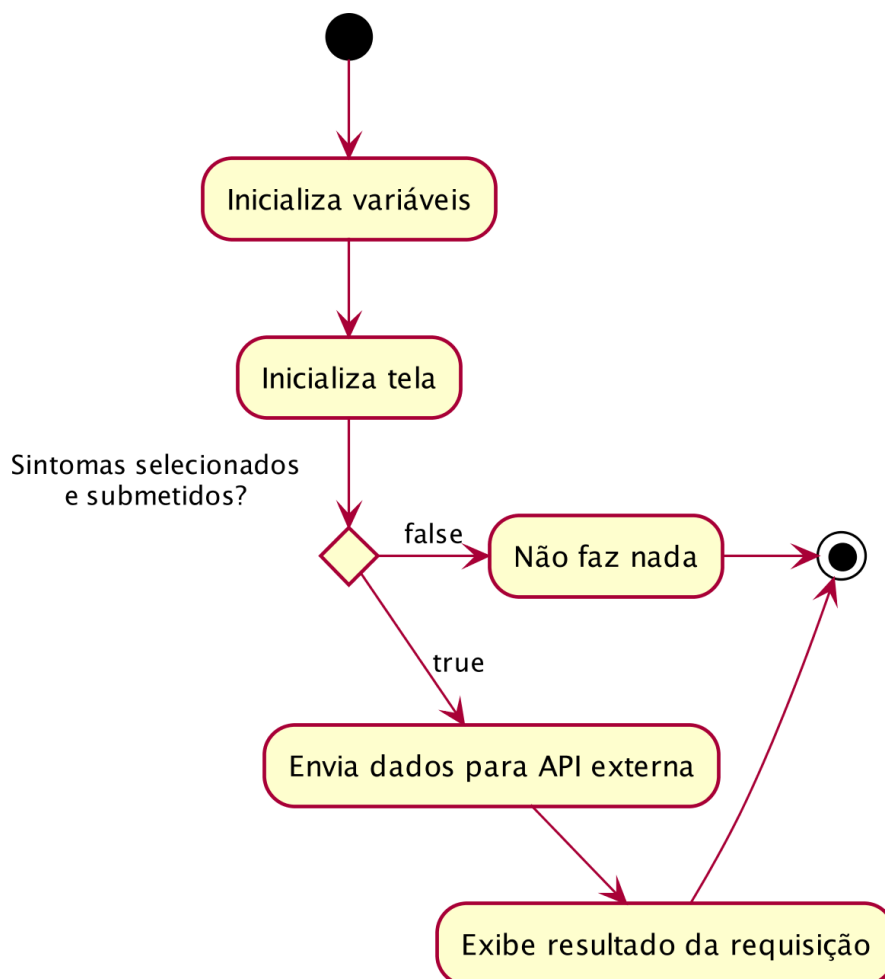
Figura 30 – Diagrama de Atividades para módulo service.dado .
