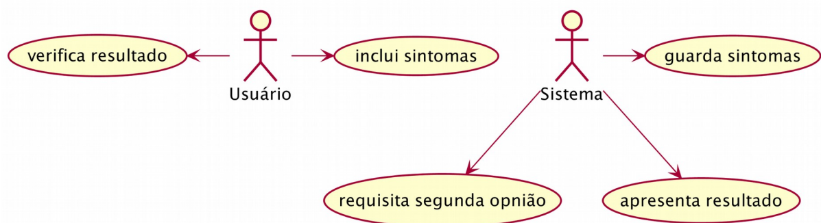
Figura 29 – Diagrama de Caso de Uso para módulo service.dado .
