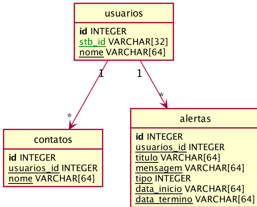
Figura 26 – Diagrama Entidade/Relação para módulo web .
