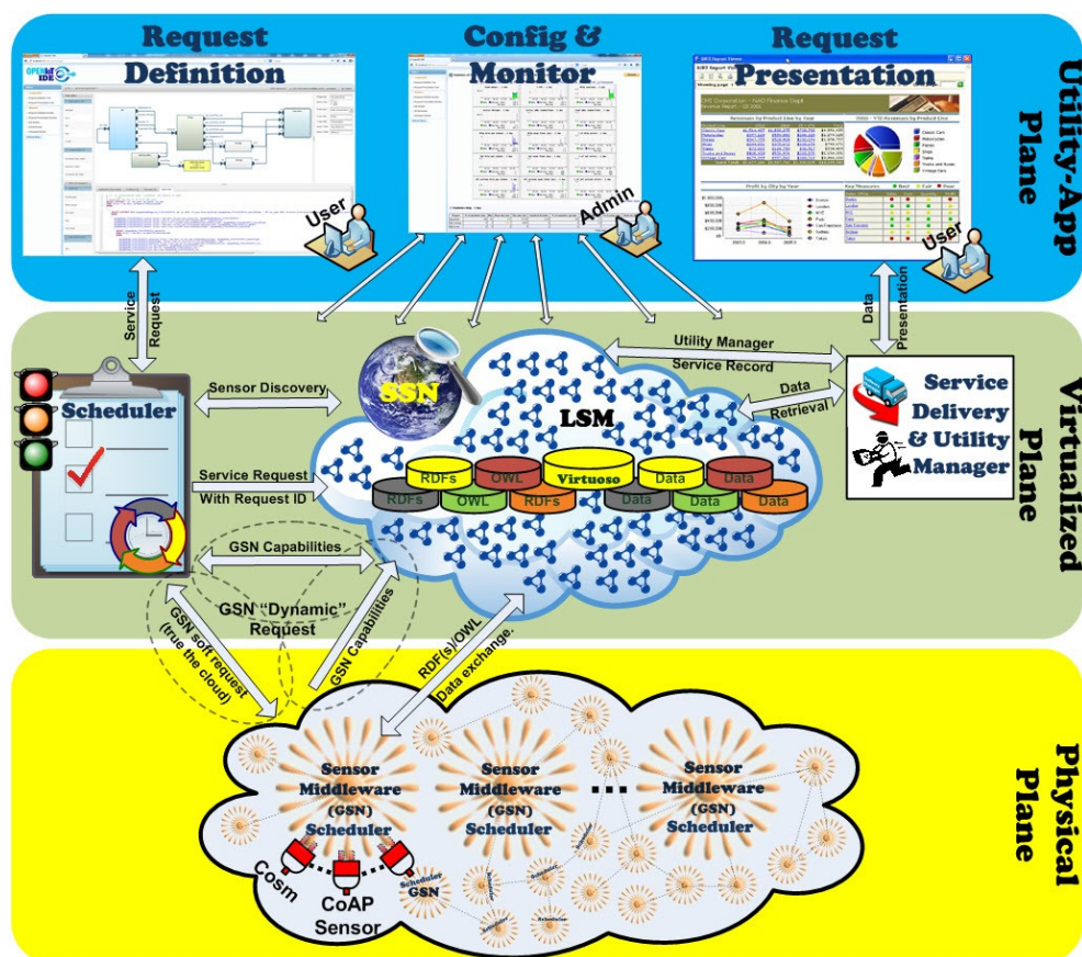
Figura 8 – Arquitetura plataforma OpenIoT
